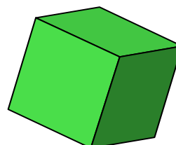
Le cube
