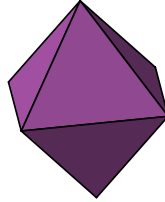
L'octaèdre
