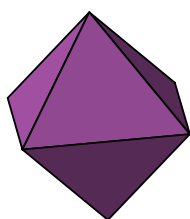
L'octaèdre
