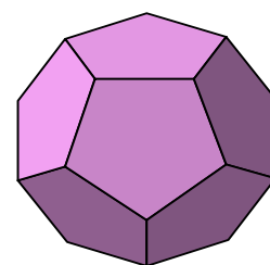
Le dodécaèdre
