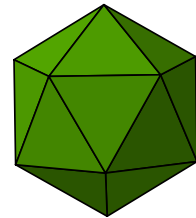
L'icosaèdre
