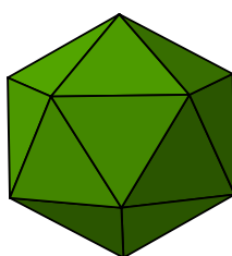
L'icosaèdre
